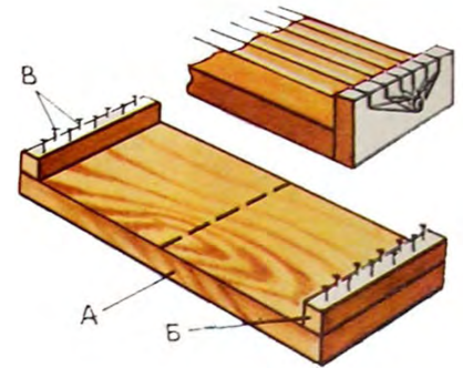
Мал. 9. А — дерев'яна дошка, Б — дерев'яний брусок, В — цвяхи
